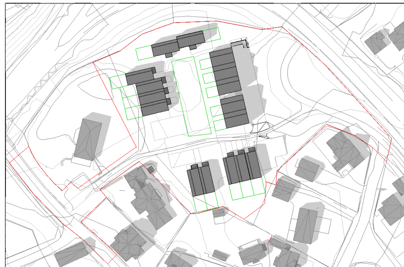
21 juni kl 15
