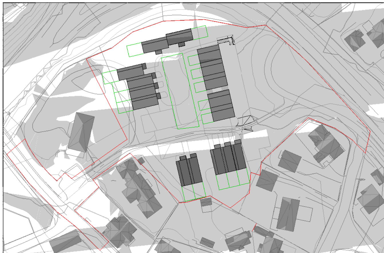
21 mars kl 18
