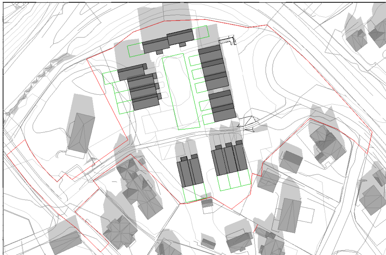
21 mars kl 12
