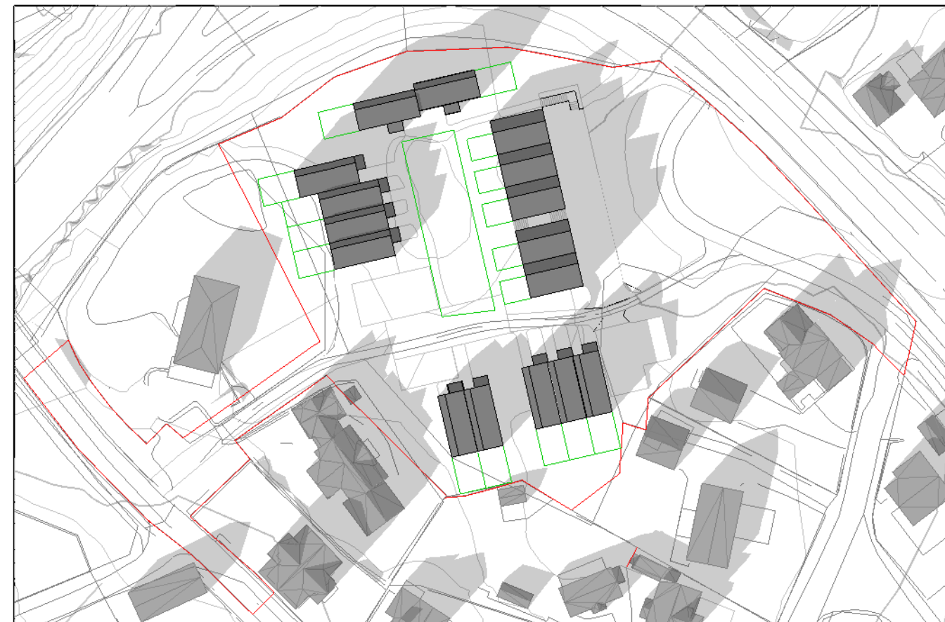
21 mars kl 15
