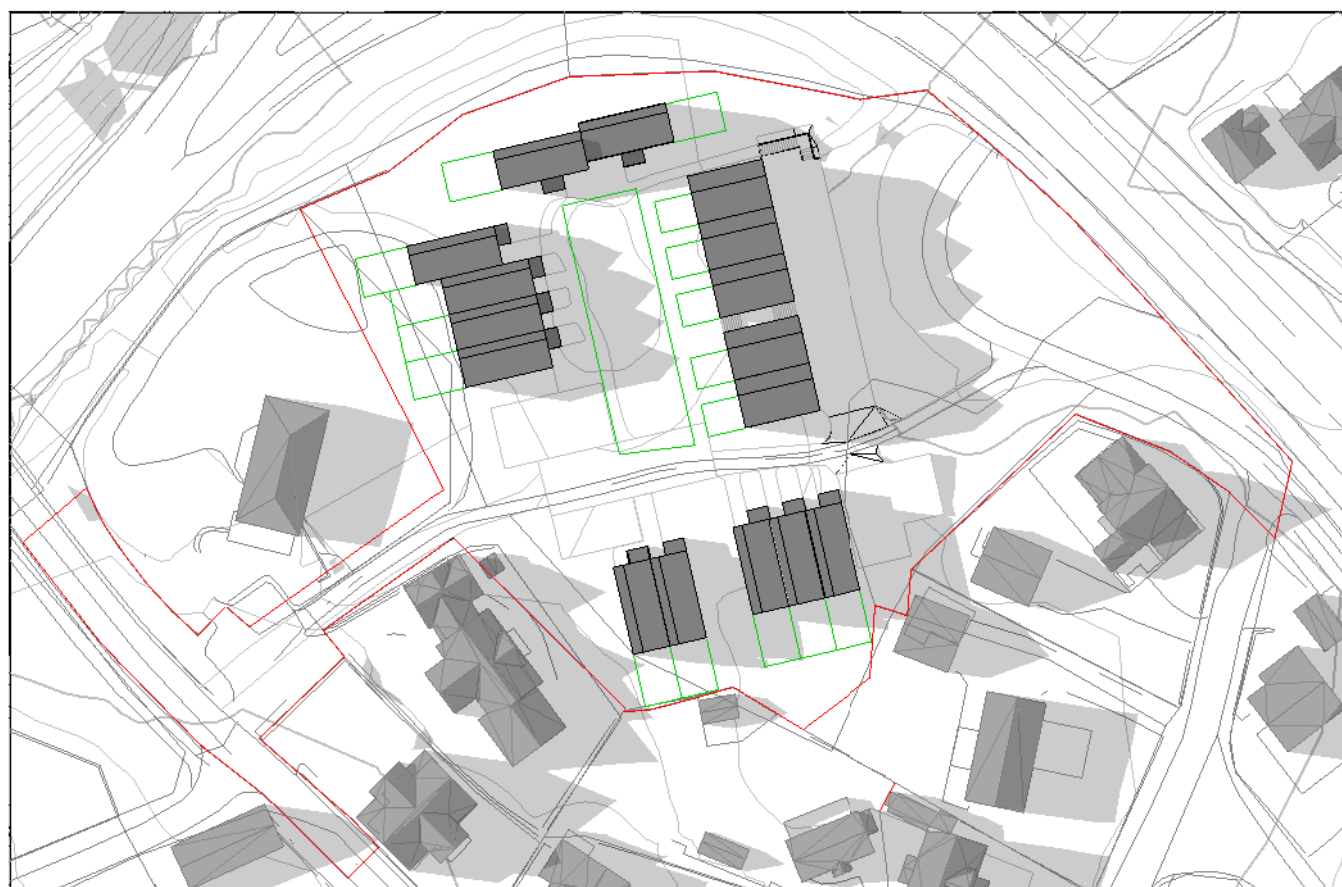
21 juni kl 18
