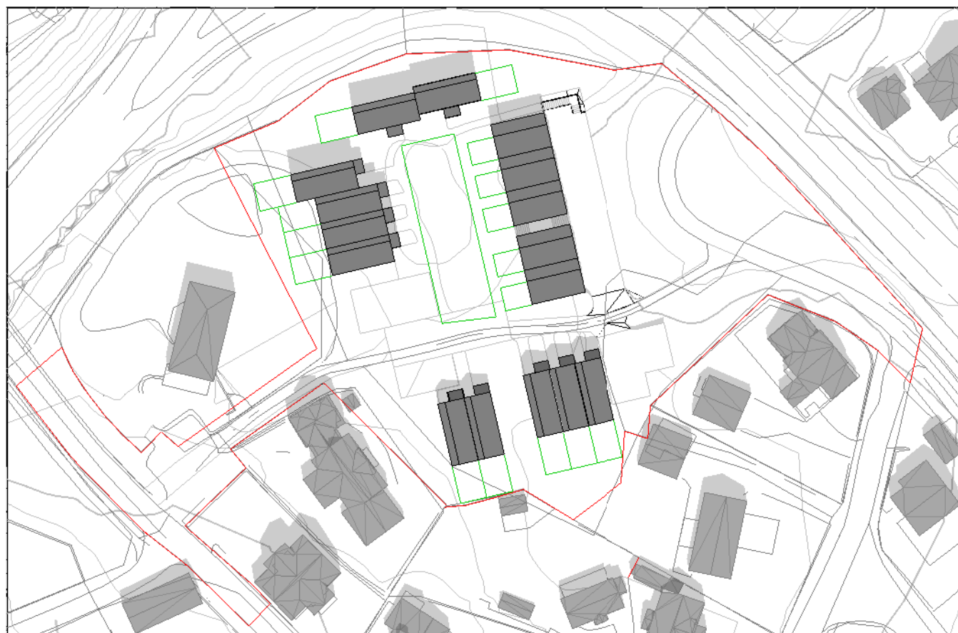
21 juni kl 12
