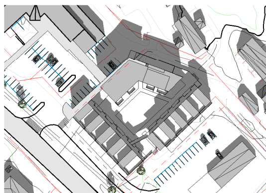
Jevndøgn kl 13 1 : 2000
